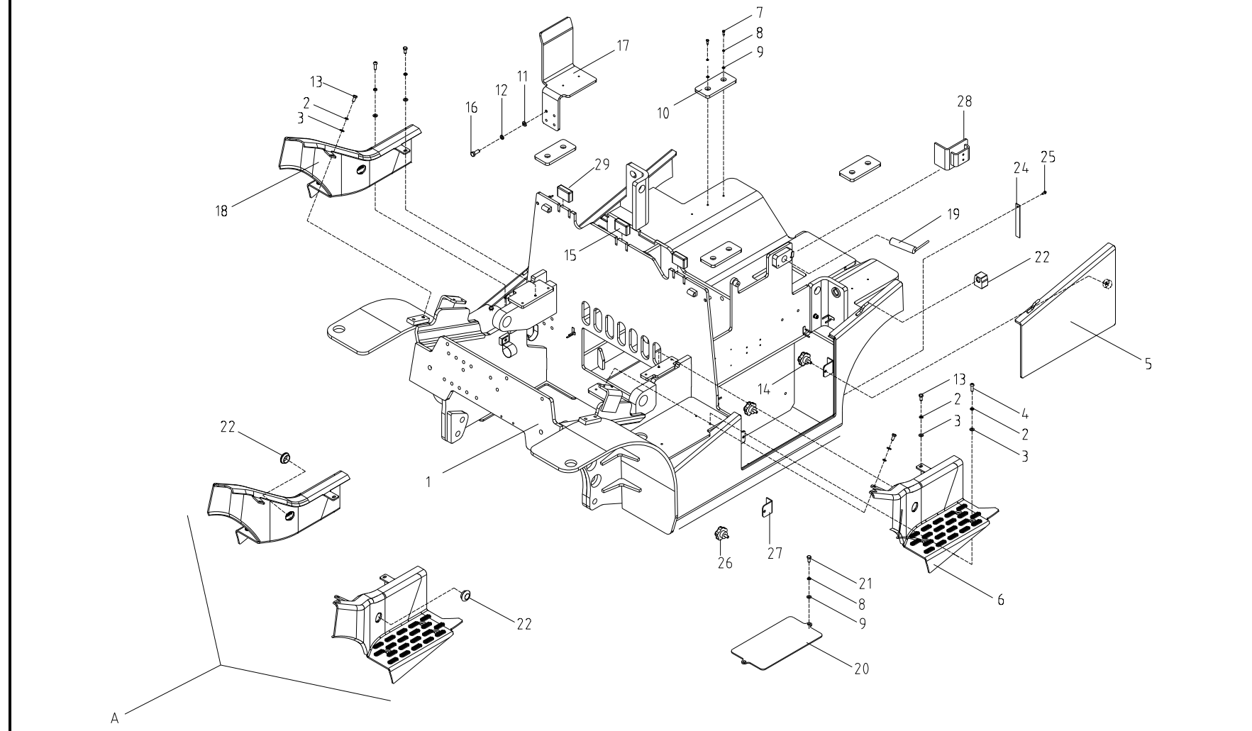
图 3-1C 车身系统 Fig.3-1C Truckbody system
