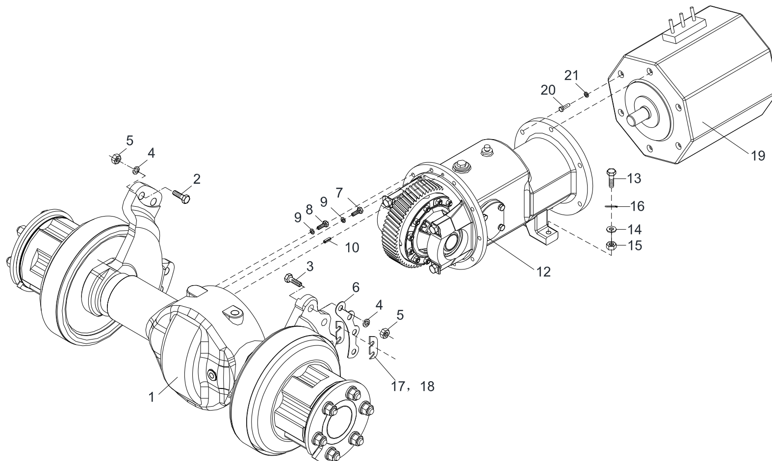
图 1-1E 传动系统 Fig.1-1E Driving system
