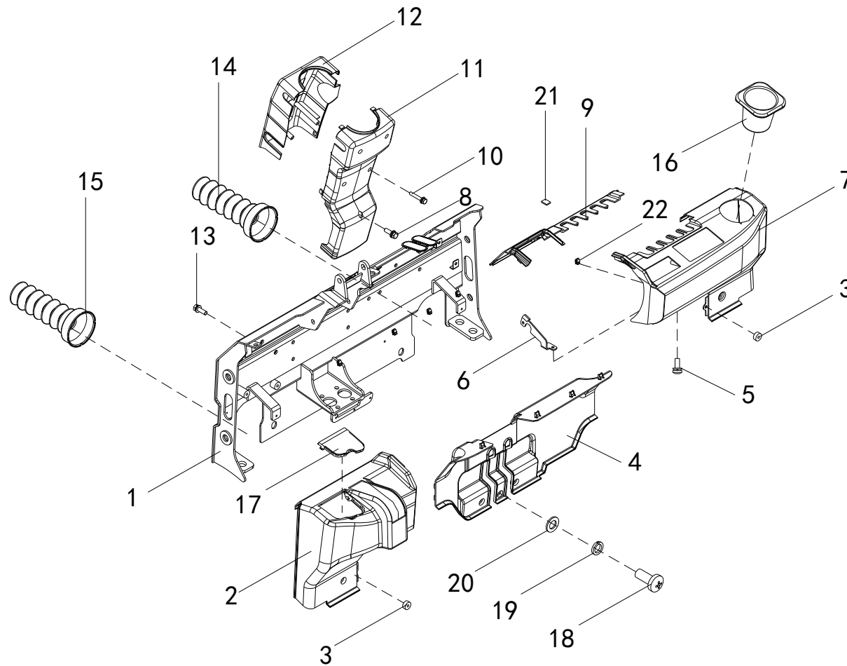
图 3-5 仪表架总成 Fig.3-5Instrument frame assy
