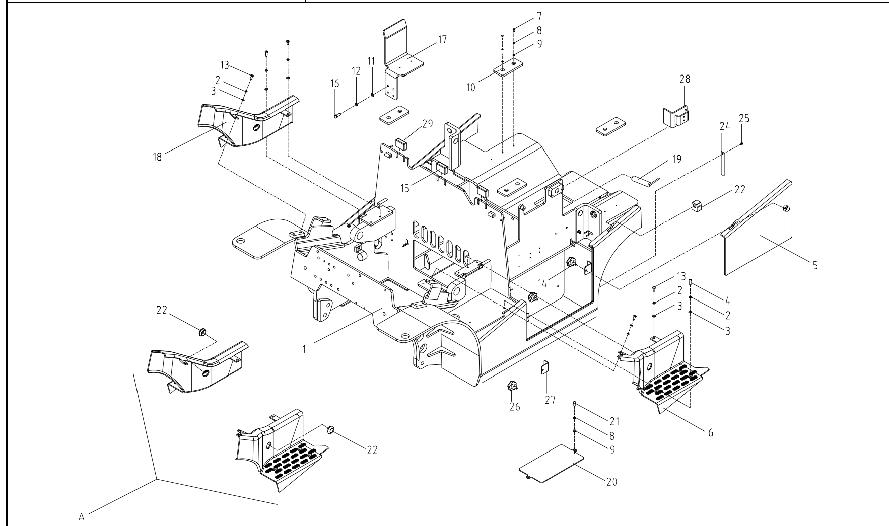
图 3-1B 车身系统 Fig.3-1B Truckbody system
