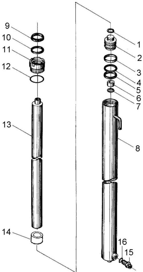
图 7 左/右升降油缸 Fig.7 Lifting cylinder,L.H. / R.H.
