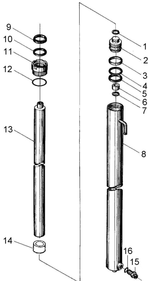
Fig.7 Lifting cylinder,L.H. / R.H.
