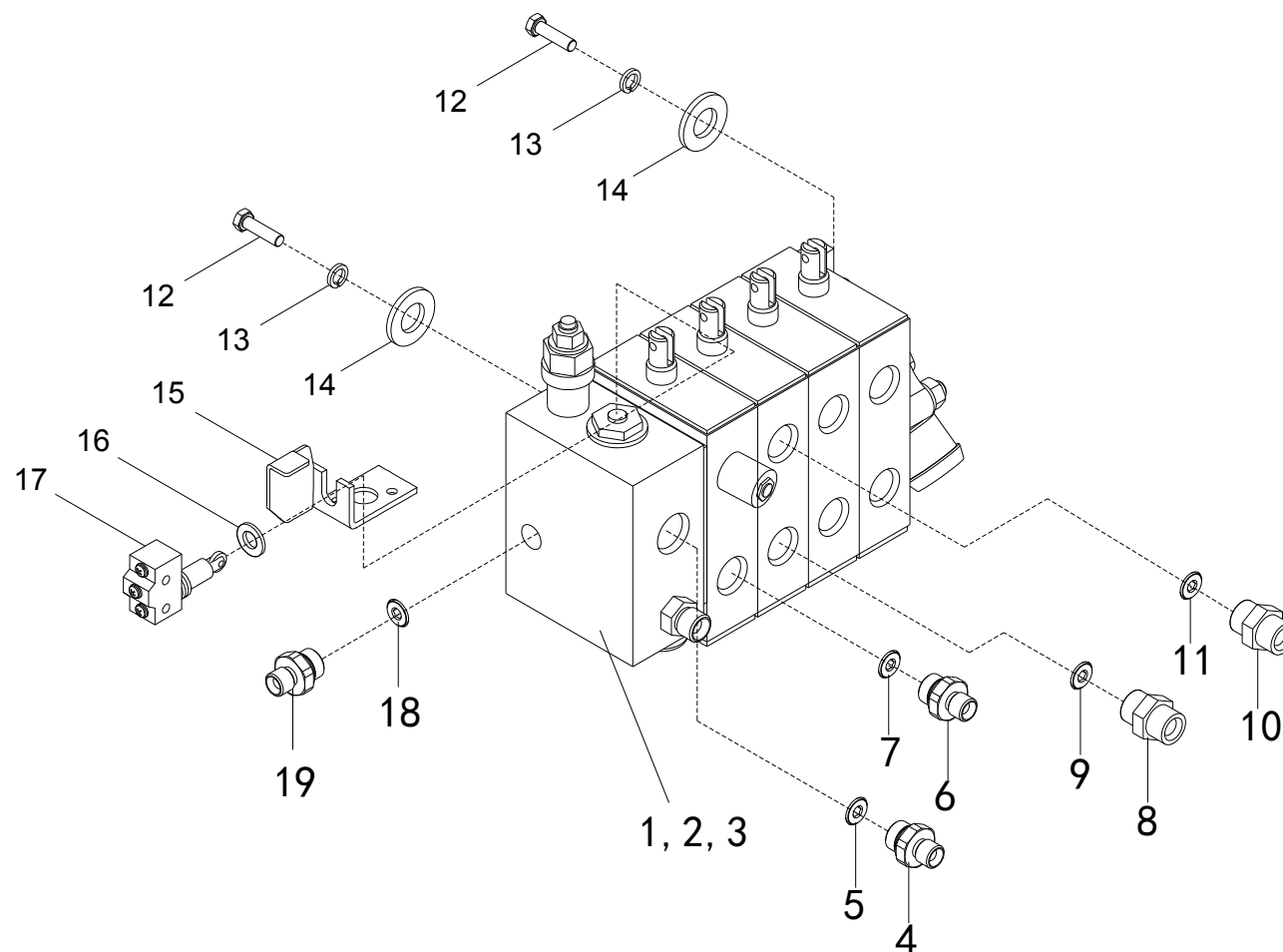
图 5-6 多路阀总成 Fig.5-6 Multi-way valve assy
