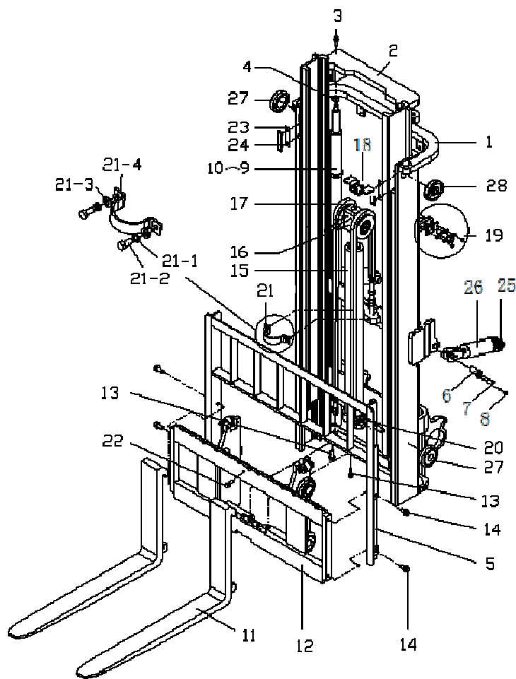
图 12 起升组件 Fig.12 Lifting part
