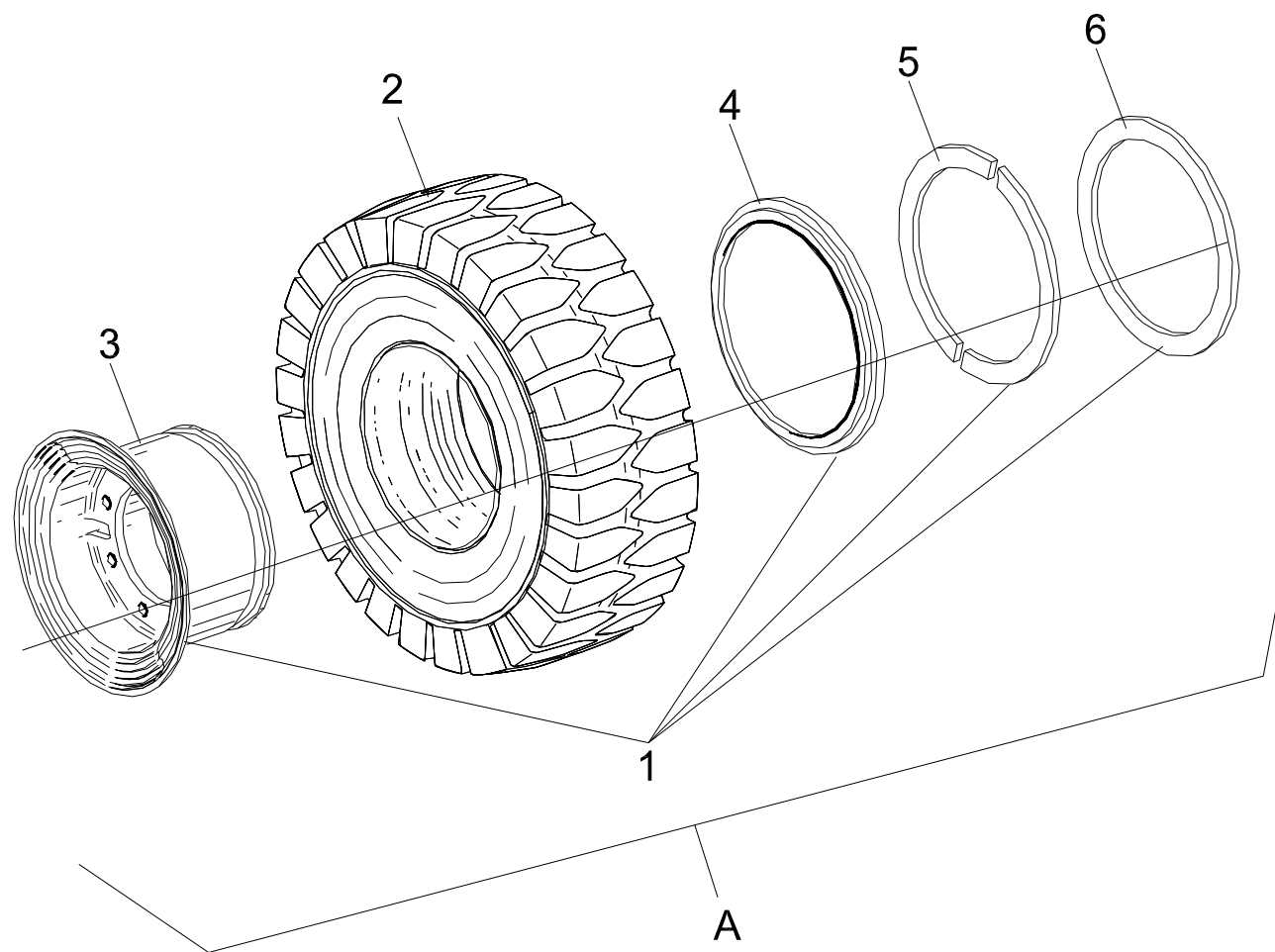
图 2-4A 后轮总成 Fig.2-4A Rear wheel assy
