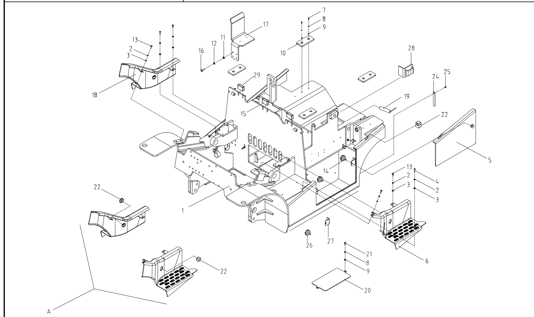
图 3-1A 车身系统 Fig.3-1A Truckbody system
